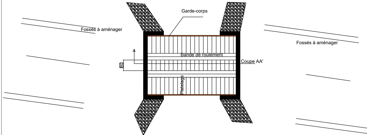
Vue en plan du Pont
